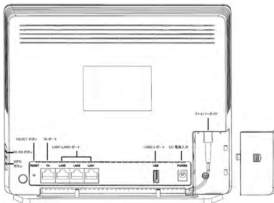
図 2-2 HG8045D 背面の外観
