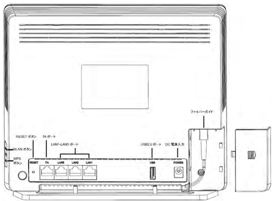
図 2-2 HG8045Q 背面の外観
